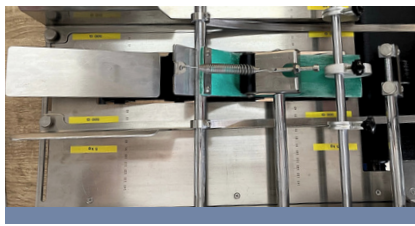
ชุดป้อนสินค้าอัตโนมัติ
